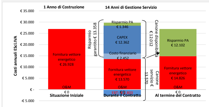
Figura 9.8 – Scenario 1: Schema di Energy Performance Contract
